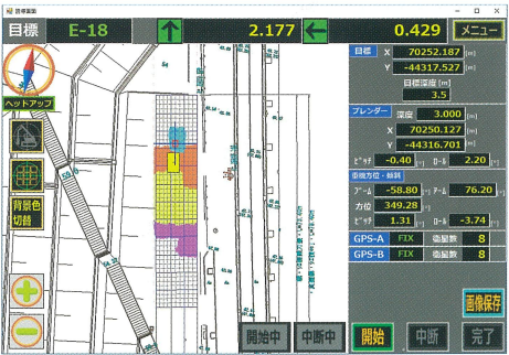
■平面誘導時管理装置表示例(施工日ごとに着色)
