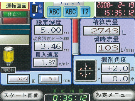
■施工管理装置「深度・流量・回転数・傾斜」
