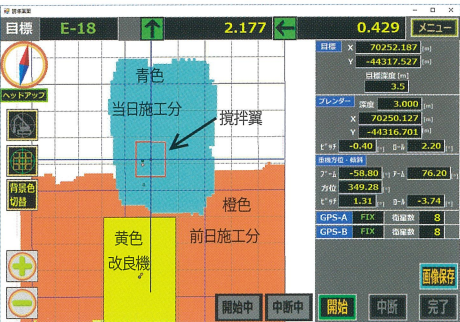
■平面誘導時管理装置表示例
